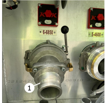
Boşaltım adaptörü
