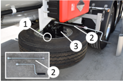
Vin tipi stepne tařıyıcısı
