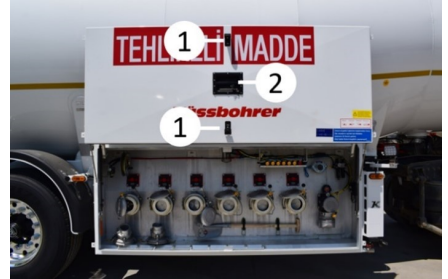
Armatür dolabı
