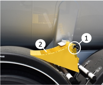
Pimli tip takoz tutucu
