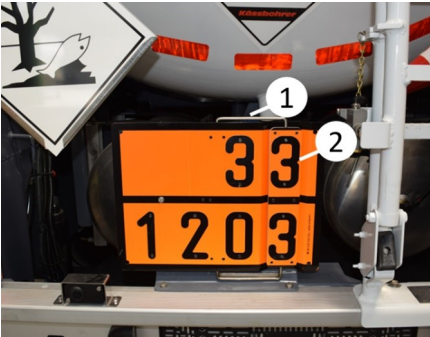
ADR plakası
