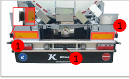
Geri yanaşma sensörleri
