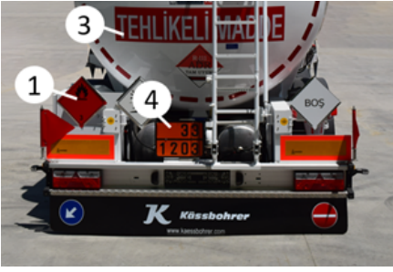
Uyarı levhası, uyarı yazısı, ADR plakası
