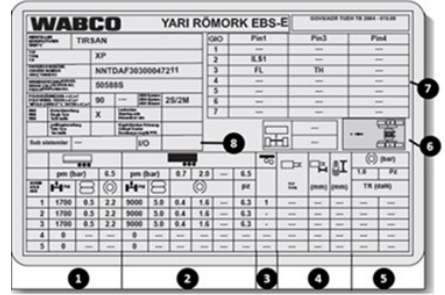
Fren etiketi
