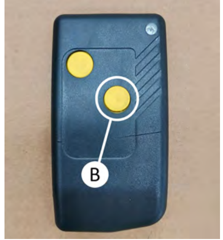
Uzaktan kumanda üzerinden brandanın açılması
