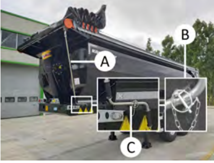
Döndürme borusunun yuvasından çıkarılması
