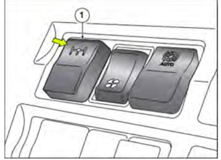
PTO düğmesinin üst konuma getirilmesi
