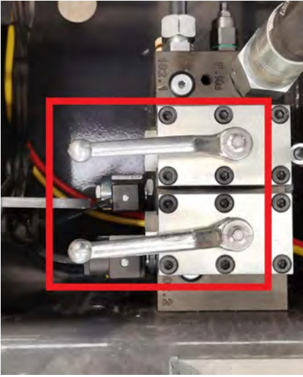
Valfin off pozisyonuna getirilmesi
