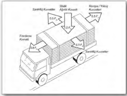
Etki eden kuvvetler
