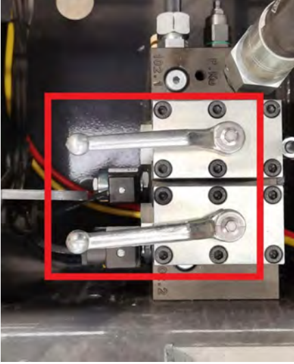
Valfin off pozisyonuna alınması
