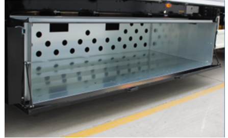
Palet dolabı açık hali
