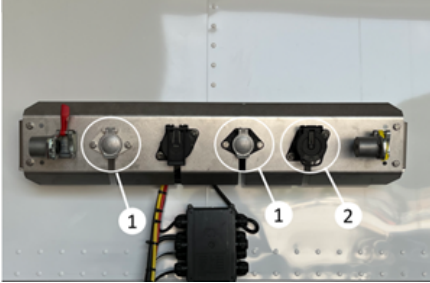
Elektrik Sistemi
