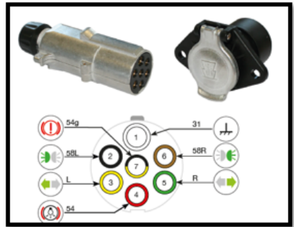
ISO 1185 Soket
