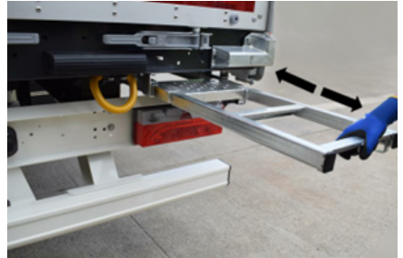
Kayar-katlanır merdiven
