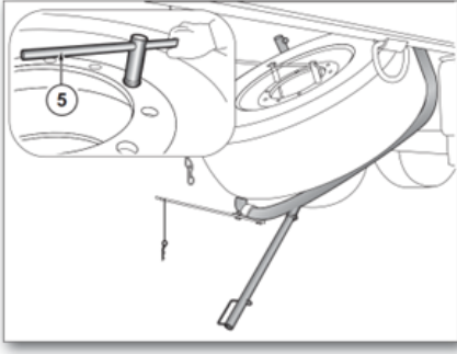
Yedek lastiği indirme
