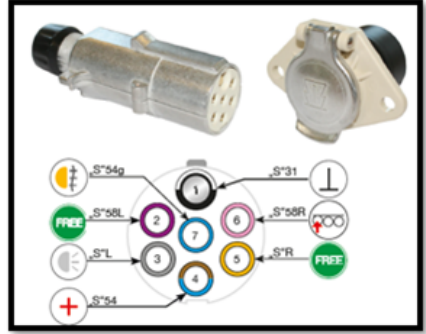
ISO3731 Soket
