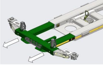
Ön uzama platformunun uzatılması
