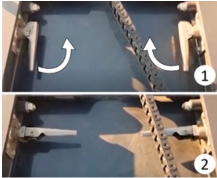
Stopper kilitlerinin açılması
