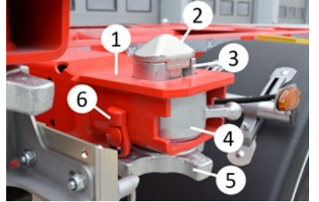
Konteyner kilidi bölümleri
