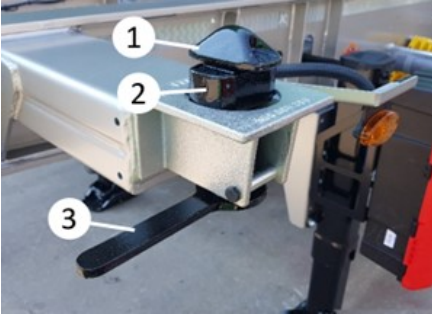
Kollu Alçalabilir Konteyner kilidi
