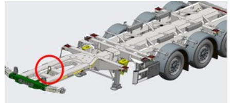
Kilit kolunun araçtaki konumu
