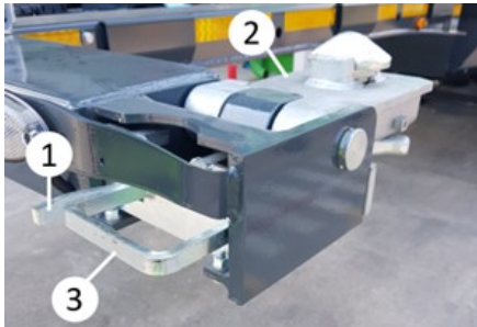
Gooseneck ön kilit
