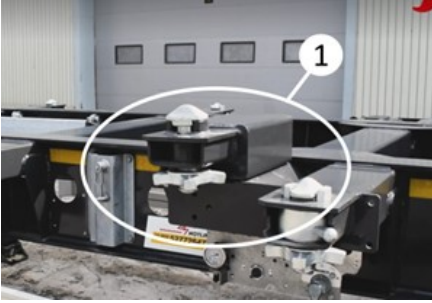
Orta katlanır kilit
