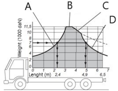
Yük dağılımı
