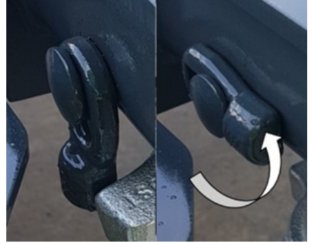
Emniyet sürüsünün 90 derece döndürülmesi
