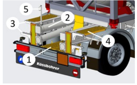
Tank konteyner taşıyıcı - arka bölge bölümleri
