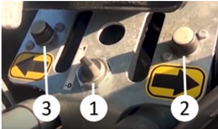
Arka uzama kontrol paneli
