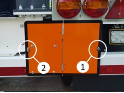
ADR plakası açık hali ve mandalları
