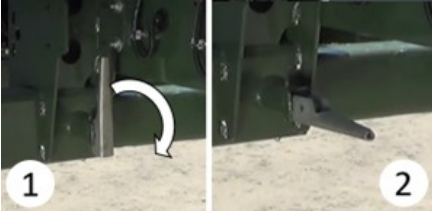
Uzar tampon kilidinin açılması
