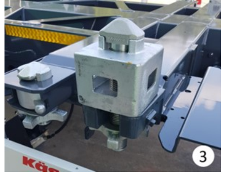
Yüksek kilidin kilit yuvasına yerleştirilmesi
