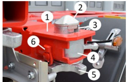
Konteyner kilidi bölümleri
