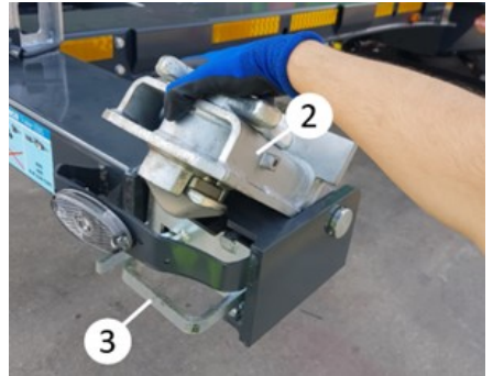
Kilidin kaldırılması
