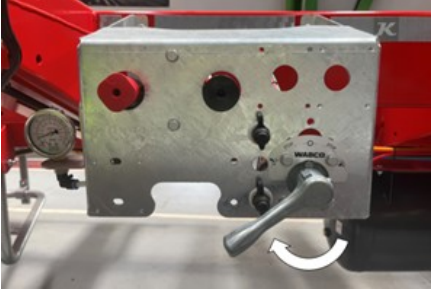
Süspansiyonun alçaltılması
