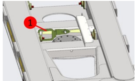
Kilit kolu
