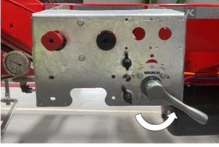
Süspansiyon yükseltilmesi
