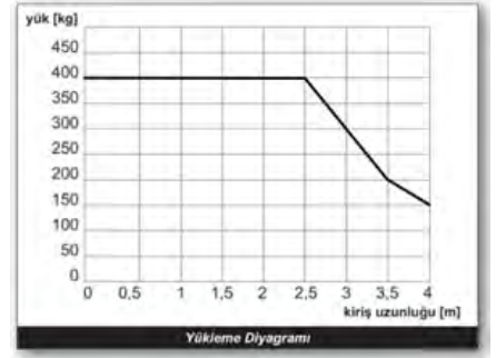
Yükleme diyagramı
