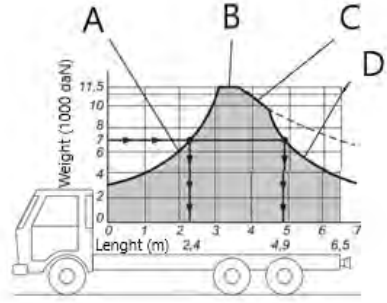
Yük dağılımı
