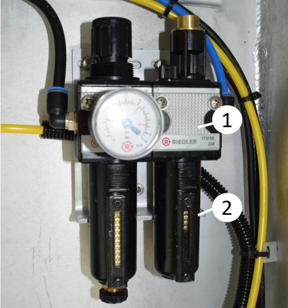
Hava şartlandırıcı ve yağ haznesi
