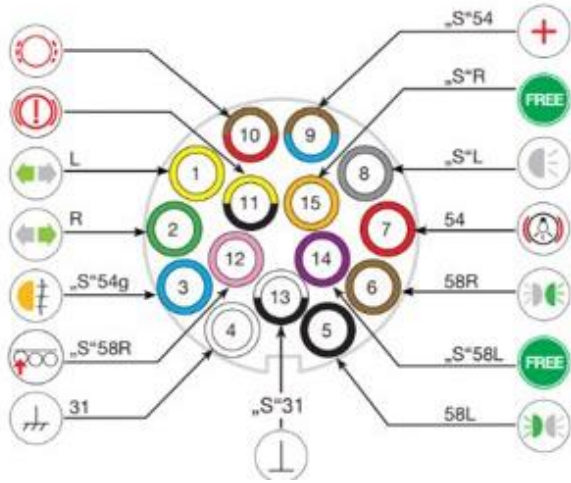
ISO 12098 Soket
