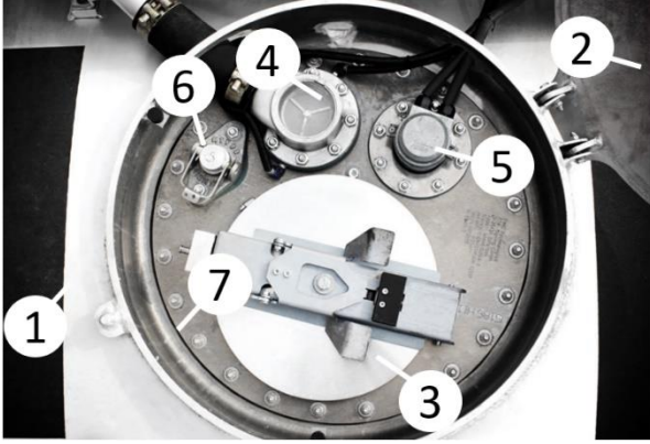
Menhol bölgesi
