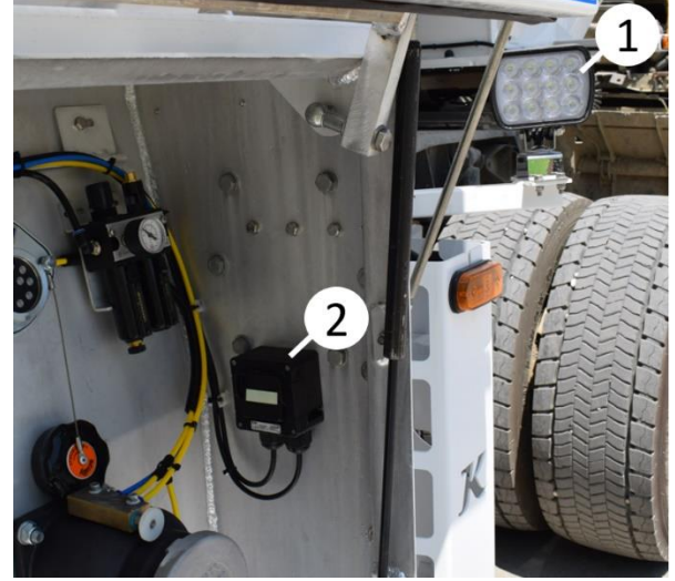
Çalışma lambası ve anahtarı
