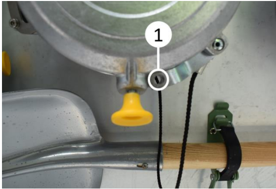
Toz kapağının mühürlenmesi
