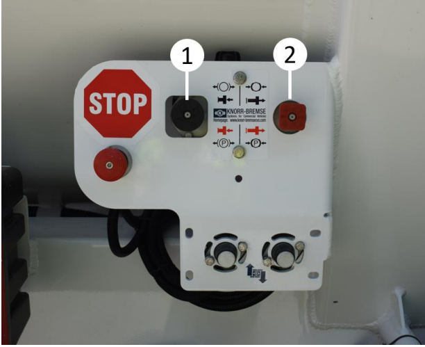
Fren kumanda elemanları
