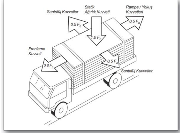
Etki eden kuvvetler
