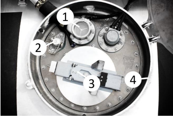
Menhol bölgesi
