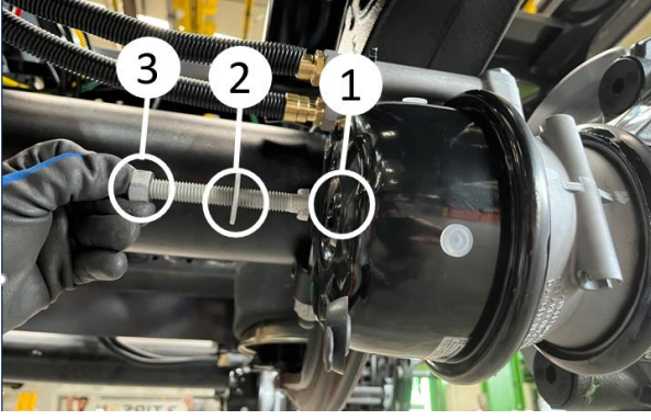
Park freninin devre dışı bırakılması
