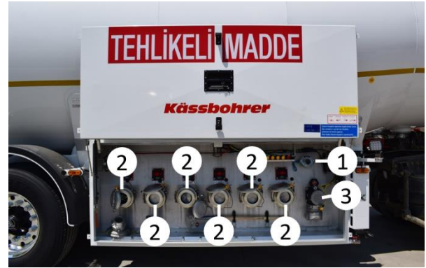
Armatür dolabı
