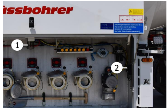
Ex-Proof lamba ve açma kapama şalteri
