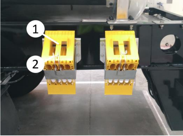
Cepli tip tekerlek takozu
