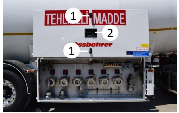
Armatür dolabı
