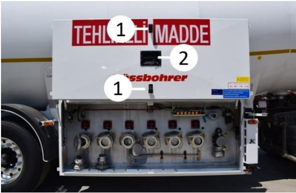
Armatür dolabı kapağı
