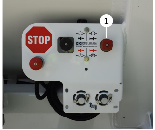
Yay yüklü park freni
