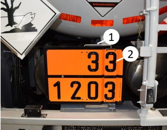
ADR plakası
