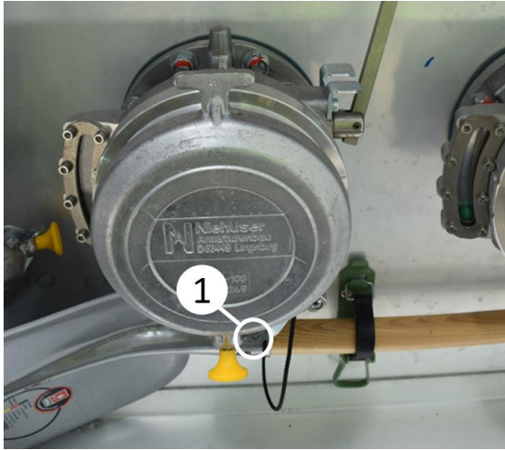
Toz kapağının mühürlenmesi
