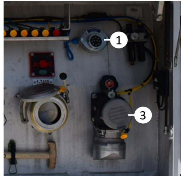
Aşırı dolum soketi, gaz geri dönüşüm
