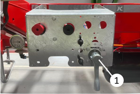
Manüel kumandalı havalı süspansiyon sürüş pozisyonu
