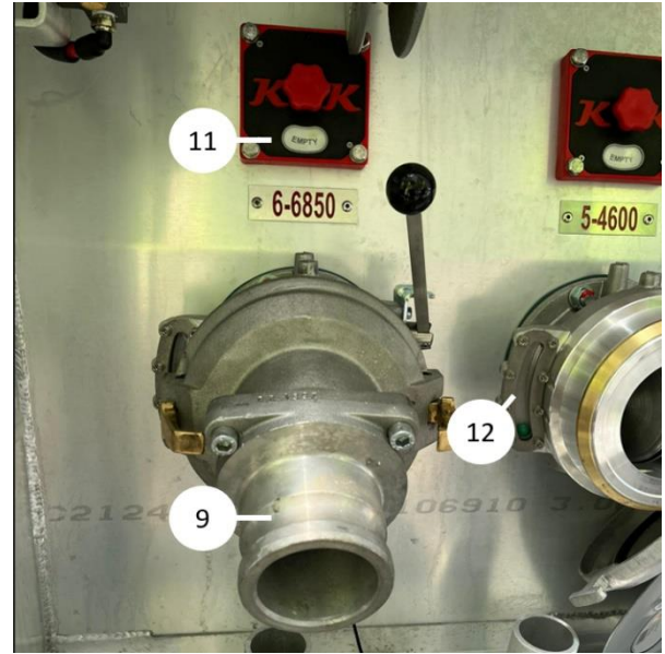
API kaplinler
