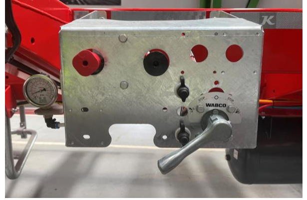
Süspansiyonun alçaltılması
