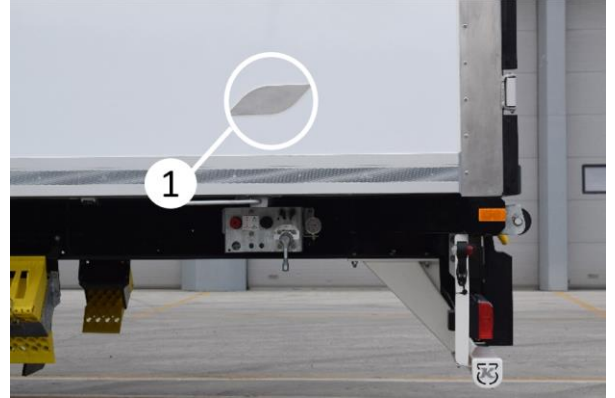
Yan panel koruma sacı
