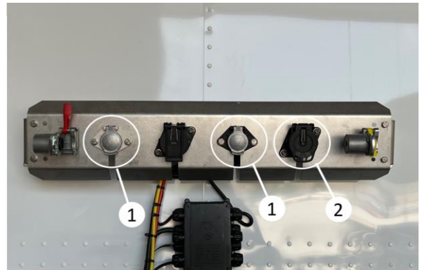
Elektrik Sistemi
