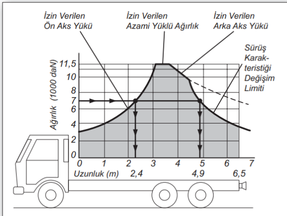
Yük dağılımı
