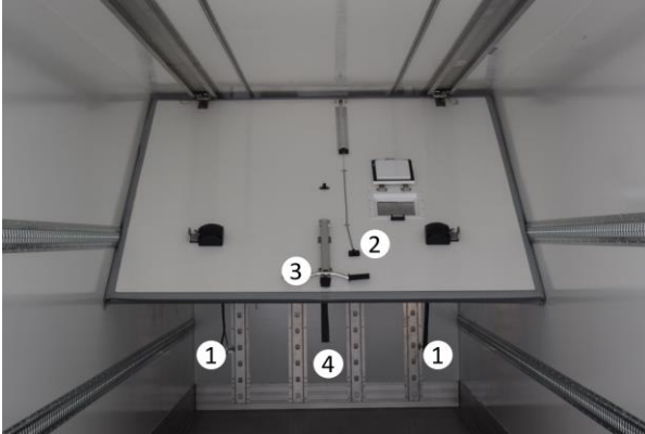
Ara bölme duvarı
