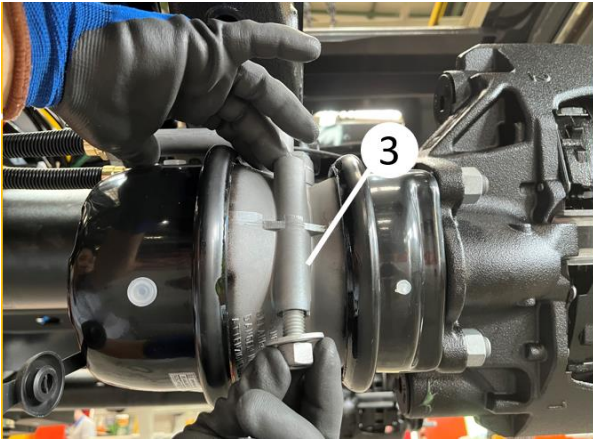
Park frenini devre dışına alma
