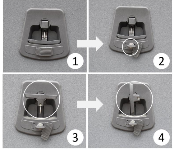
Alternatif dolap kilidinin açılması
