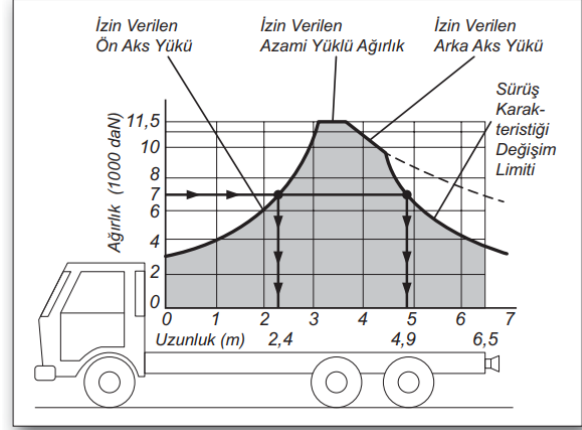
Yük dağılımı
