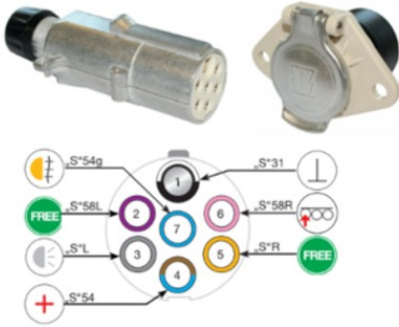
ISO 3731 Soket
