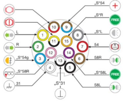
15 Pinli Soket
